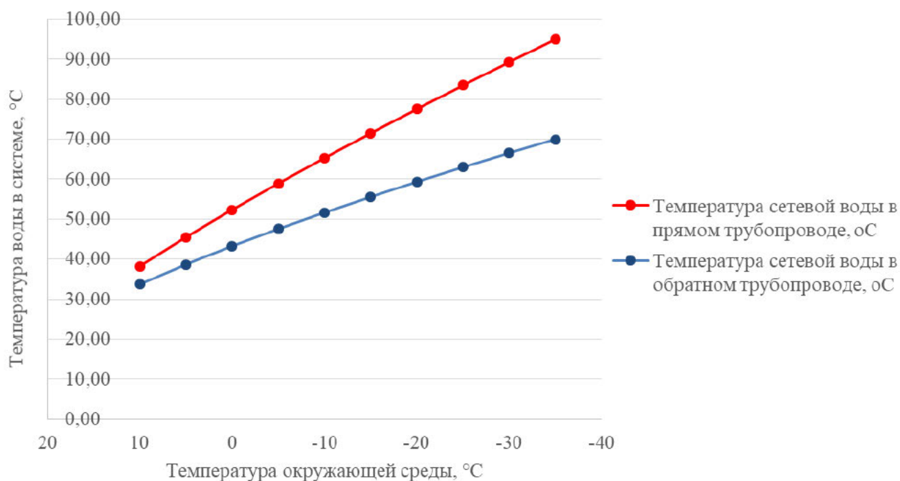
Рисунок 2.2 – График изменения температур теплоносителя (температурный график 95/70°С)
