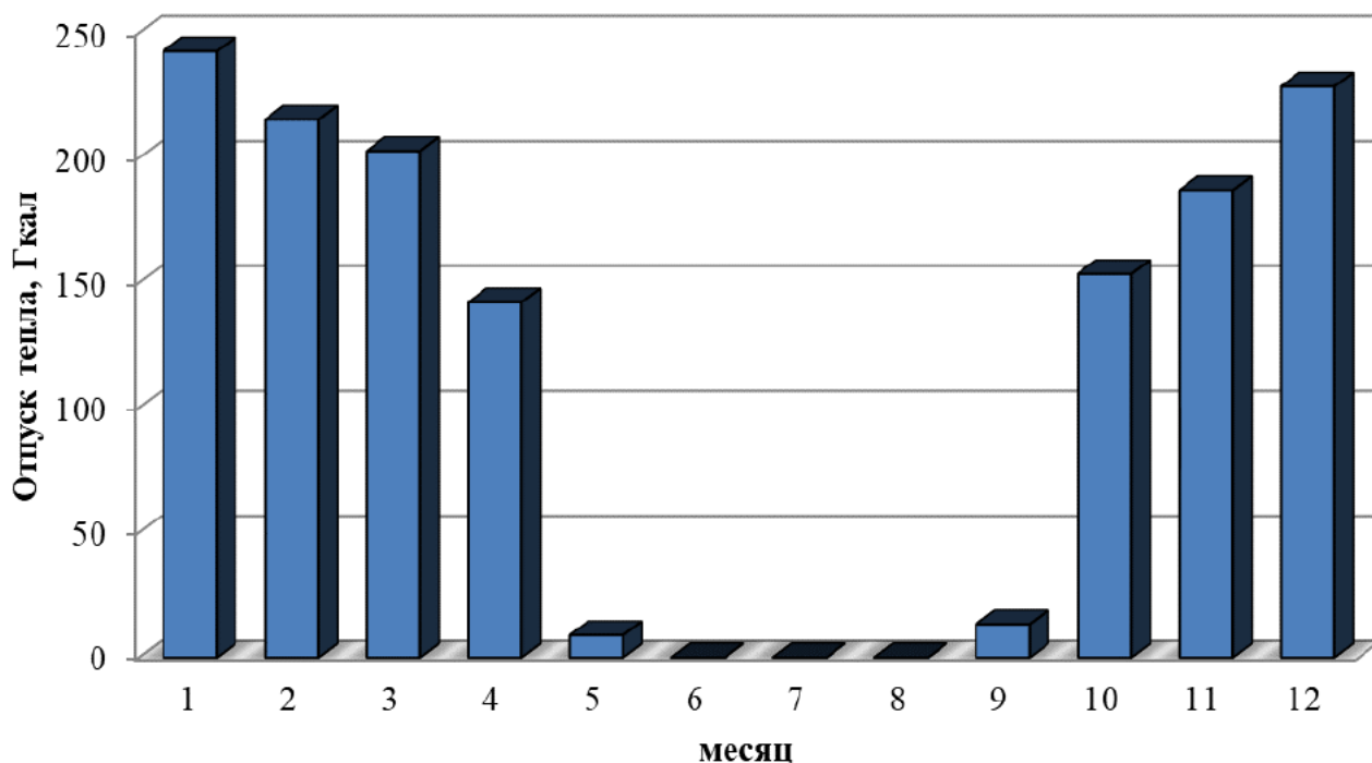
Рисунок 1.2 – Оптимальный температурный график отпуска тепловой энергии для котельной с. Бородиновка
