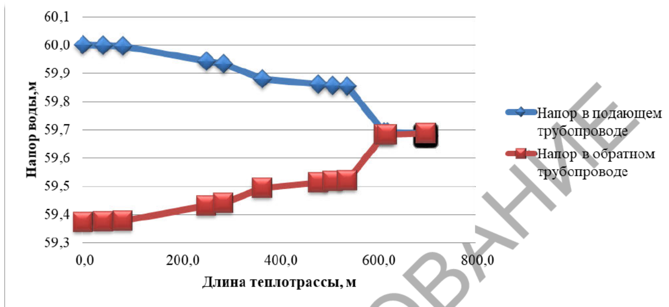
Рисунок 2.3 – Пьезометрический график тепловой сети котельной с. Бородиновка по магистральному выводу
