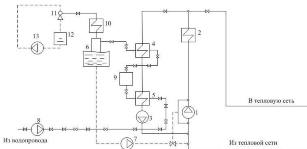
Рисунок 2.1 – Принципиальная тепловая схема котельной с водогрейными котлами: 1 - сетевой насос; 2 - водогрейный котел; 3 - рециркуляционный насос; 4 - подогреватель
