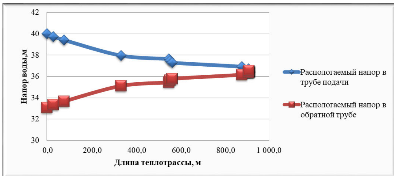
Рисунок 2.3 – Пьезометрический график тепловой сети поселковой котельной по магистральному выводу
